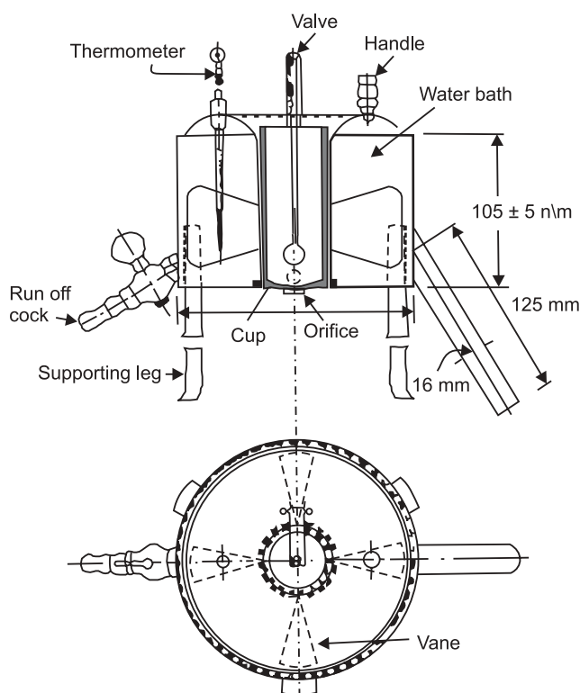
Fig. 18.4 Tar Viscometer
