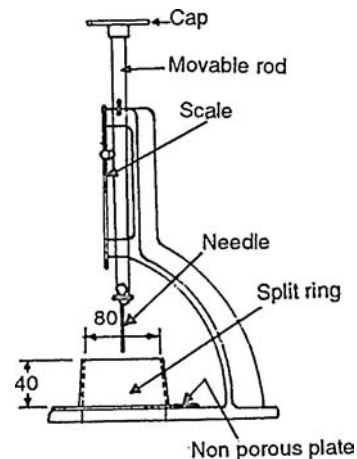
Fig. 5.9 Vicat's Apparatus
