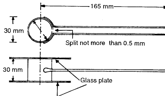
Fig. 5.10 Le-chatelier Apparatus
