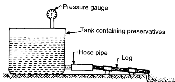
Fig. 4.6 Boucherie Process
