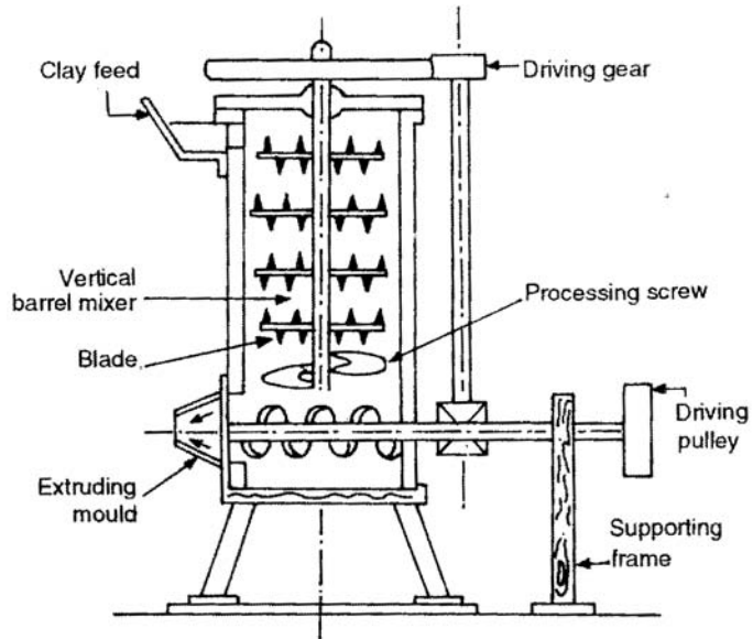
Fig. 2.3 Pug Mill
